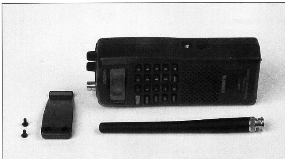
Figuur 4 (links): De aanpassing van de antenne-ingang op 145 MHz.
