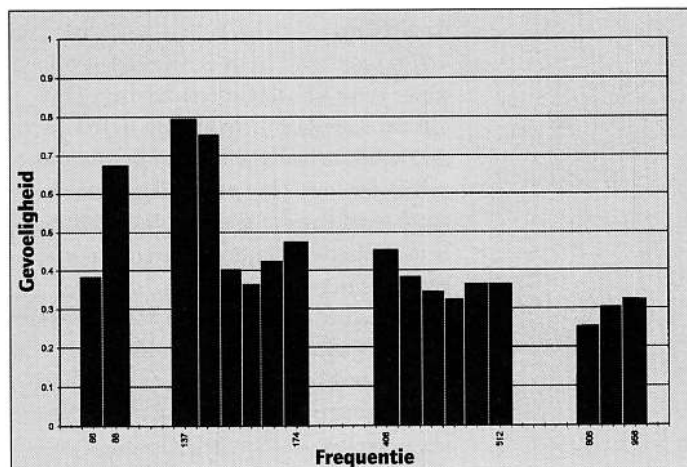
Figuur 1: De gevoeligheid van de COM 115.
